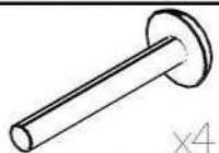
x4 Screw - M8 L40 - Internal hexagon D6
